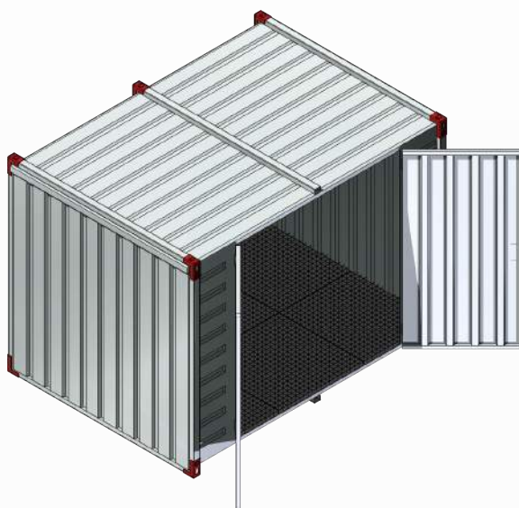
Milieucontainer met roostervloer, lekbak en 2 ventilatieroosters, dubbele deuren zijwand
