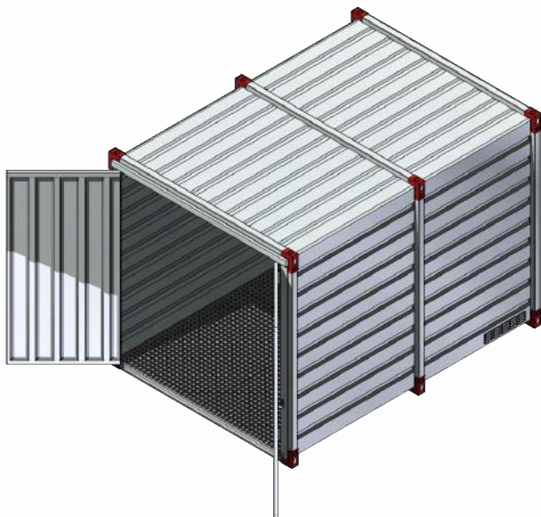
Milieucontainer met roostervloer, lekbak en 2 ventilatieroosters, dubbele deuren kopzijde
